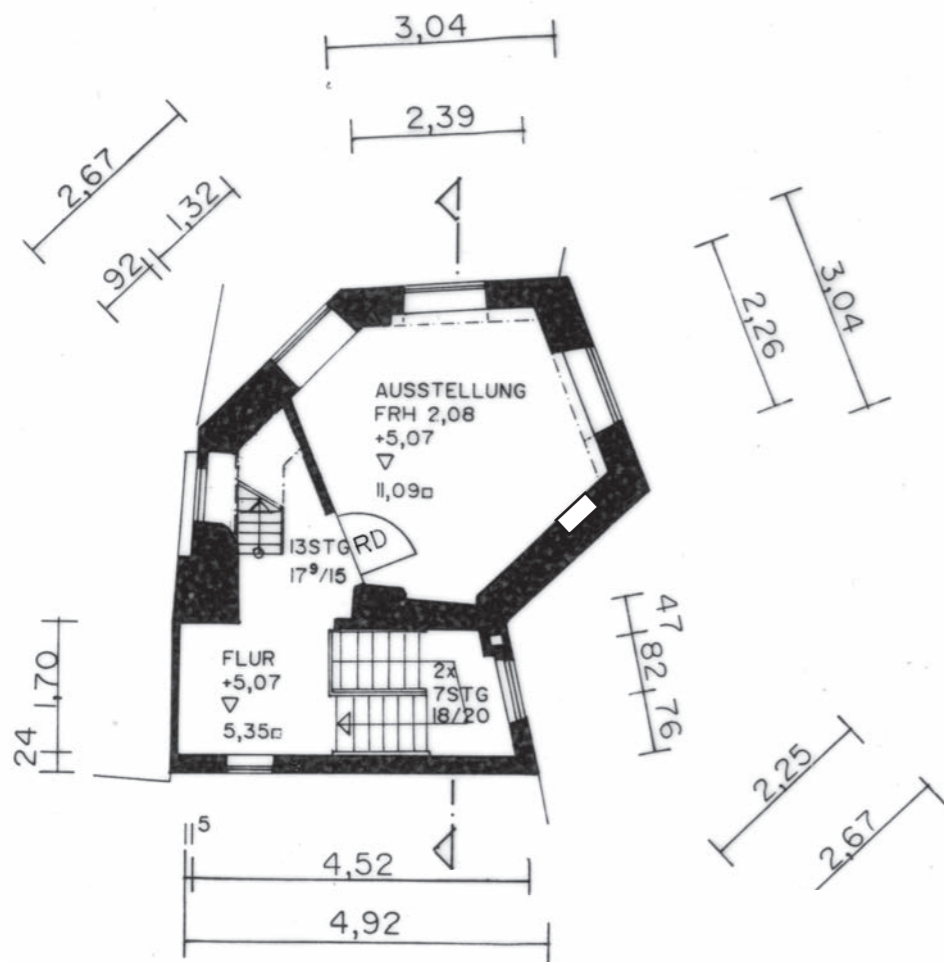
2. Obergeschoß
