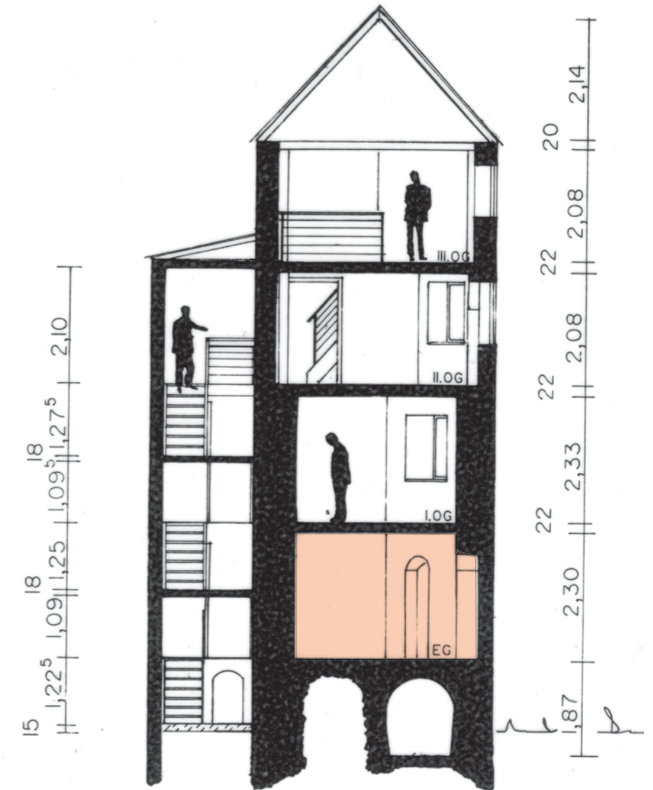
Schnitt
