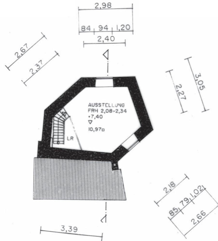
3. Obergeschoß
