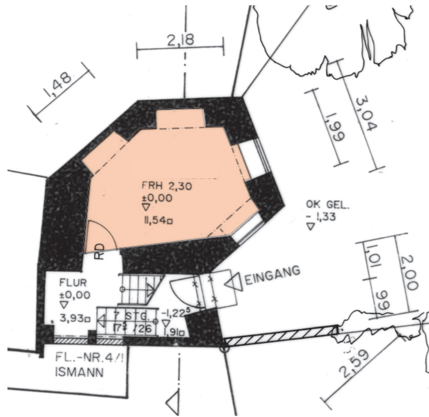
Erdgeschoß
